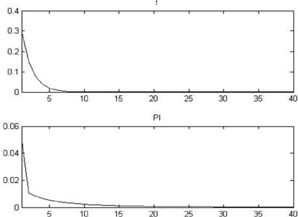
نمودار (۳): تغییرات نقدینگی و تورم بر اثر بروز شوک نفتی
