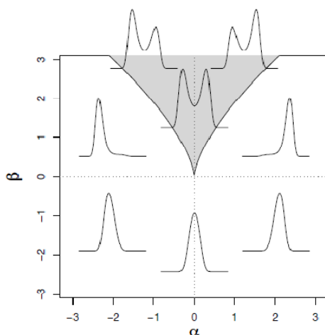
شکل ۳- تابع چگالی کاسپ در نواحی مختلف صفحه کنترل
